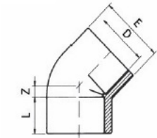
Kolano 45°
