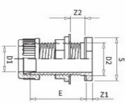
Śrubunek zbiornika z nakrętką zaciskową GZ
