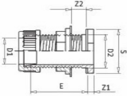
Śrubunek zbiornika z nakrętką zaciskową GZ
