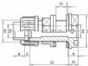
Śrubunek zbiornika ze złączką KW
