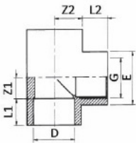
Trójnik 90° KW x KW x GW
