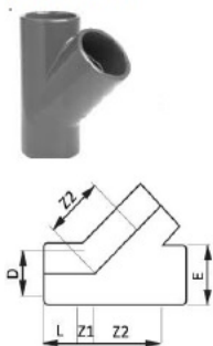
Trójnik 45°
