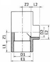
Trójnik redukcyjny 90° KW x KW x KW
