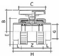
Zawór kulowy BVD
