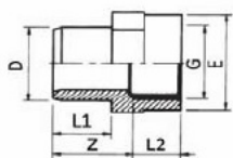
Złączka KZ x GW
