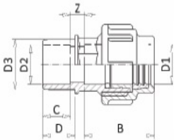
Złączka KW x KZ x PE
